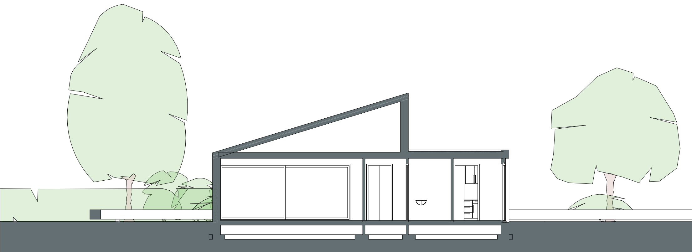
Doorsnede B-B
