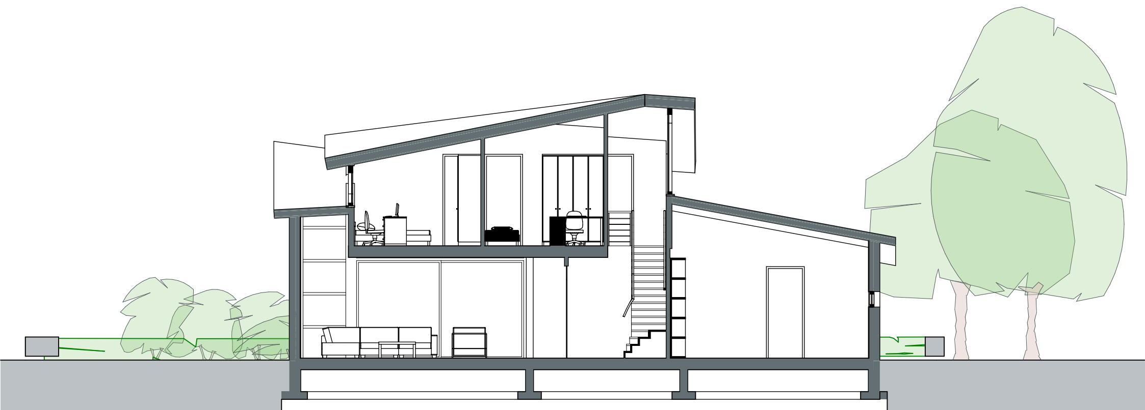
Doorsnede B-B
