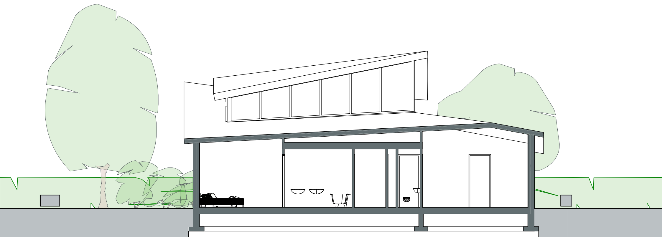
Doorsnede A-A
