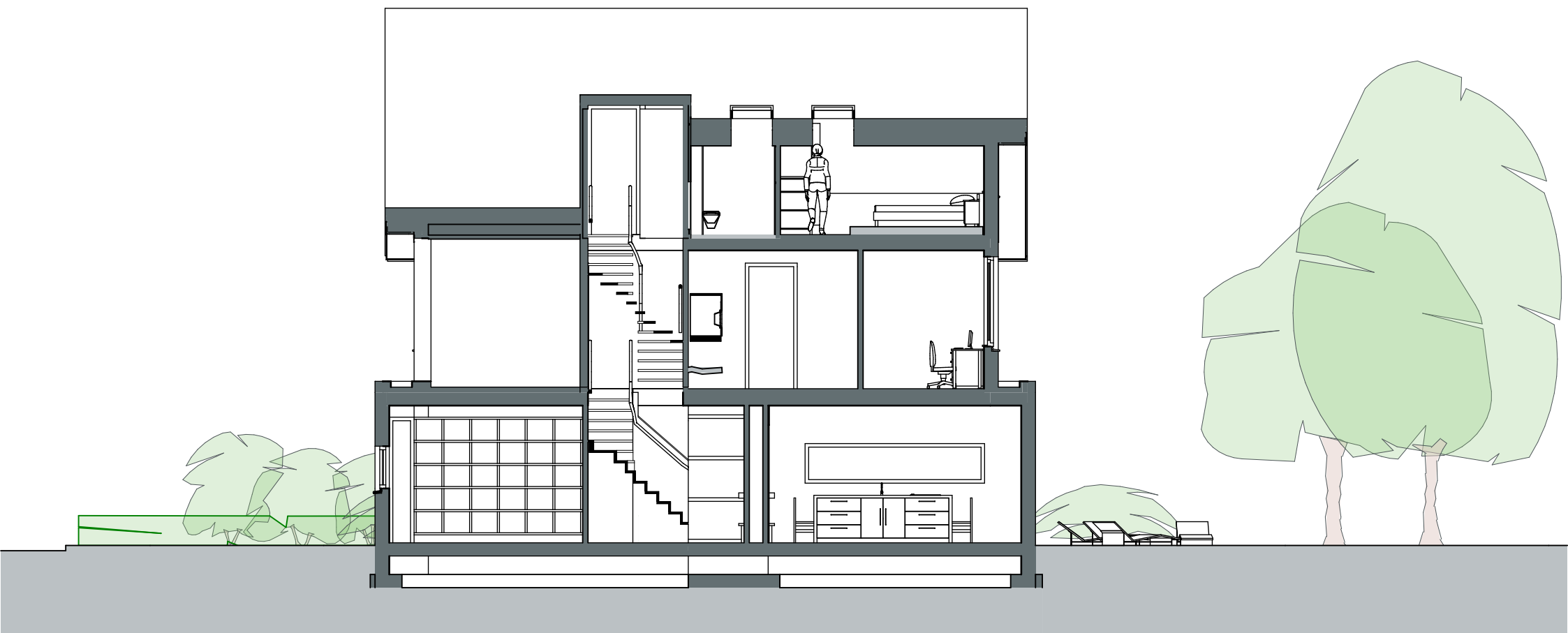
Doorsnede B-B
