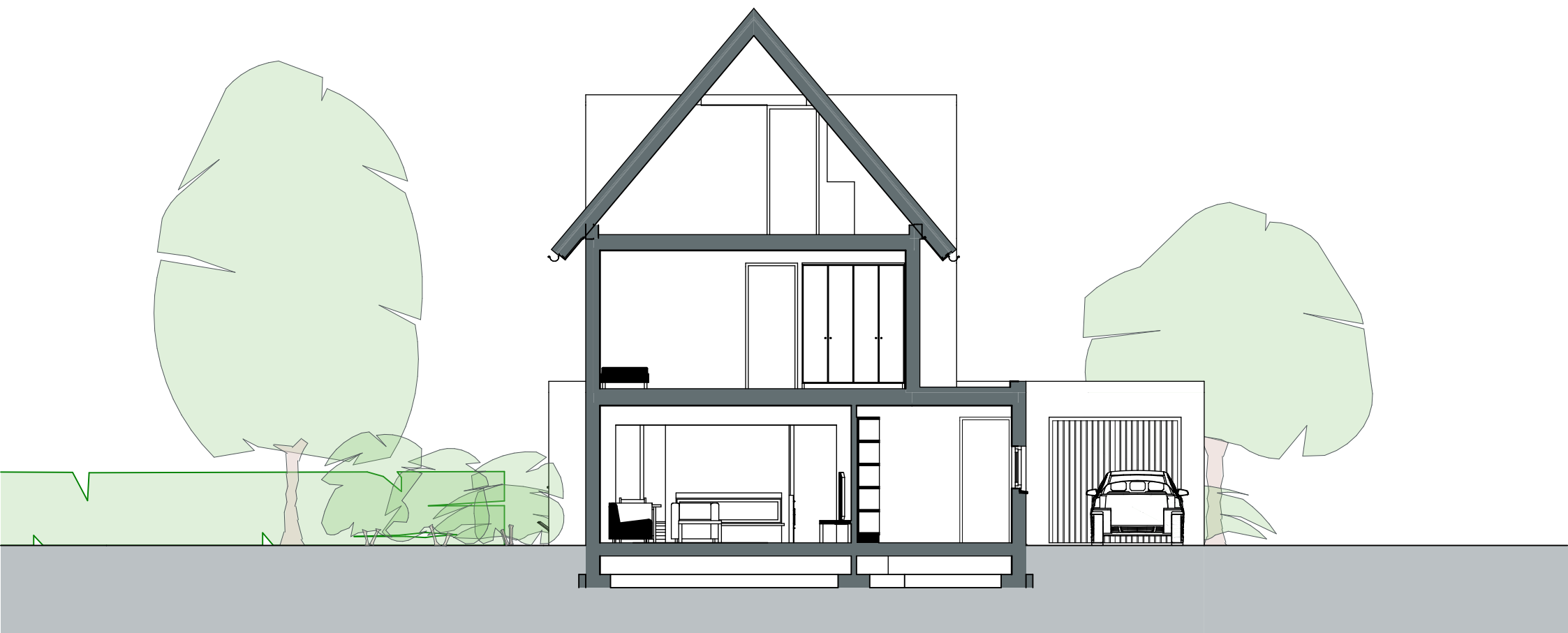
Doorsnede A-A
