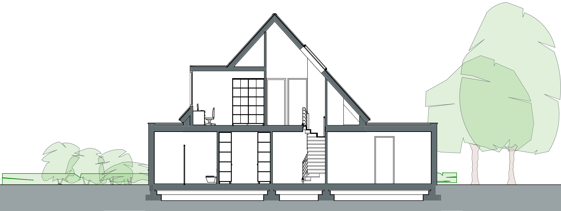
Doorsnede B-B
