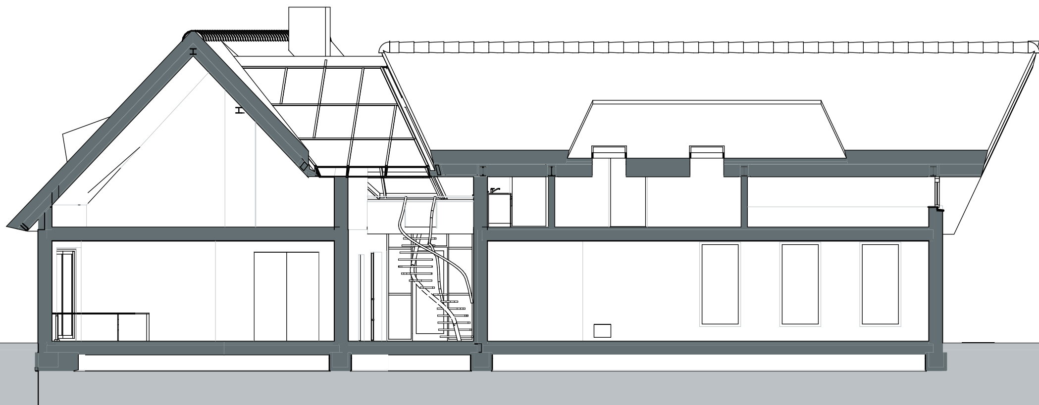
Doorsnede B-B
