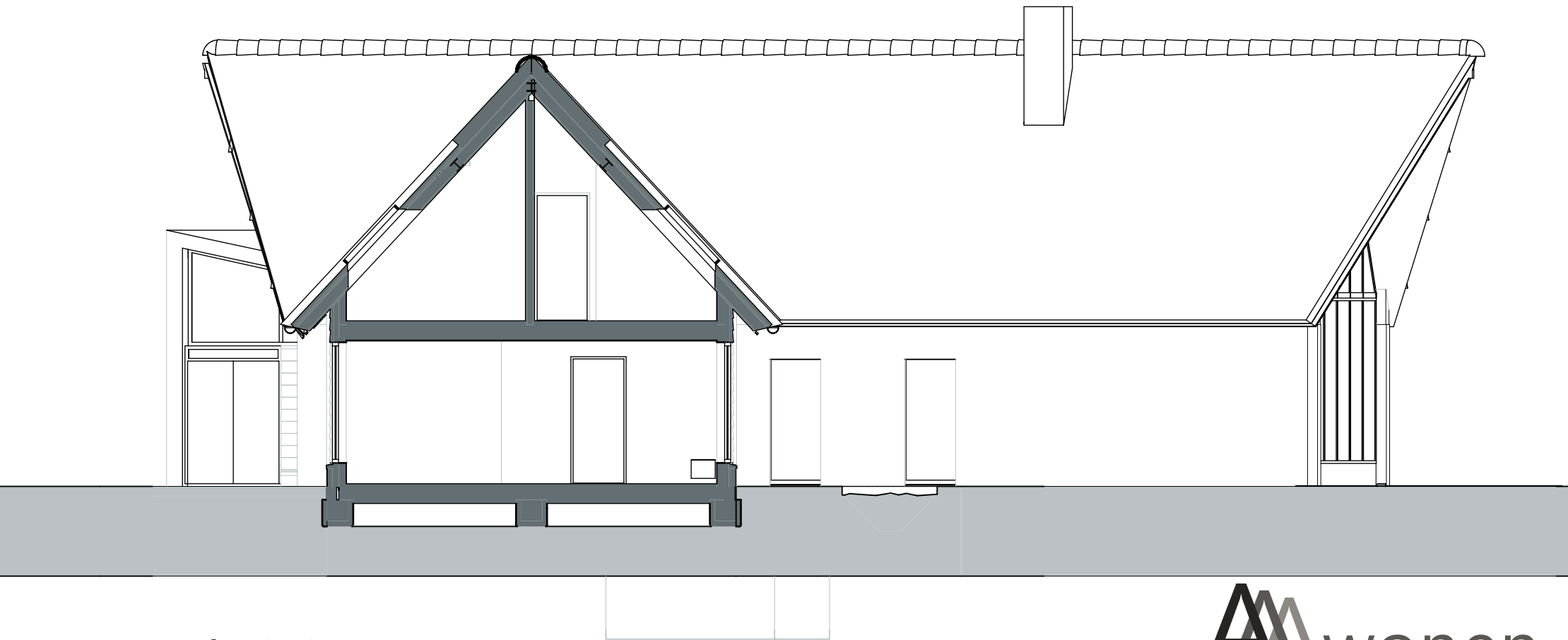
Doorsnede A-A
