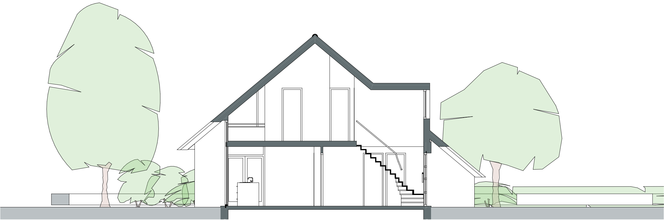
Doorsnede A-A
