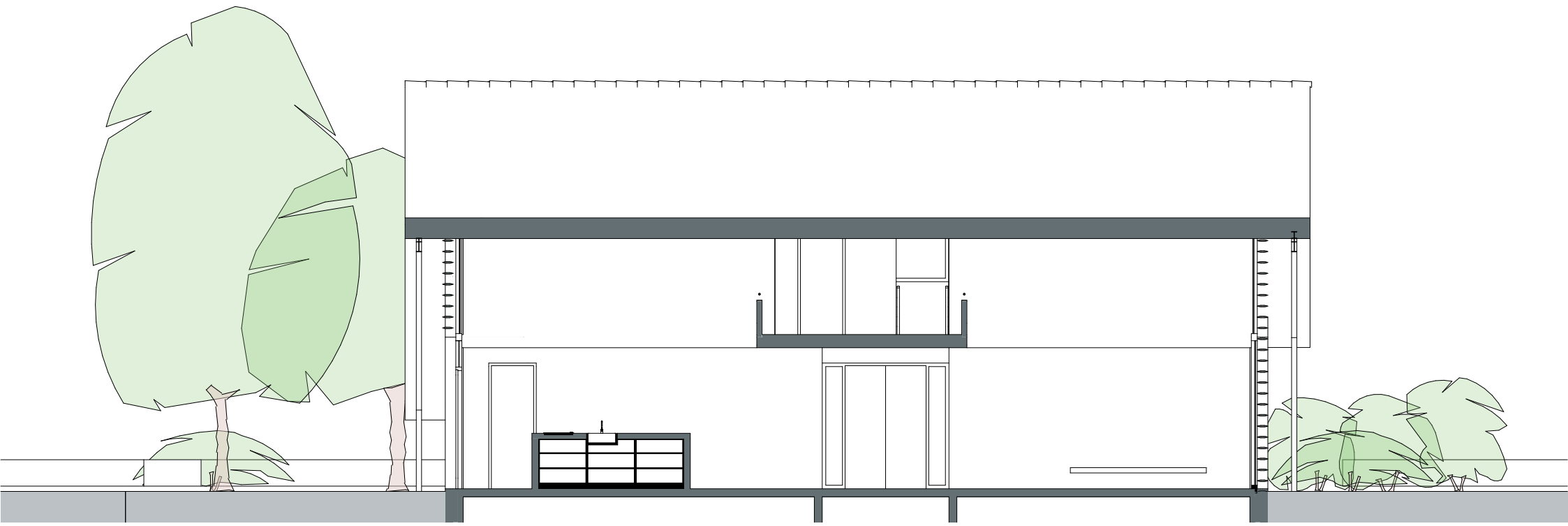
Doorsnede B-B
